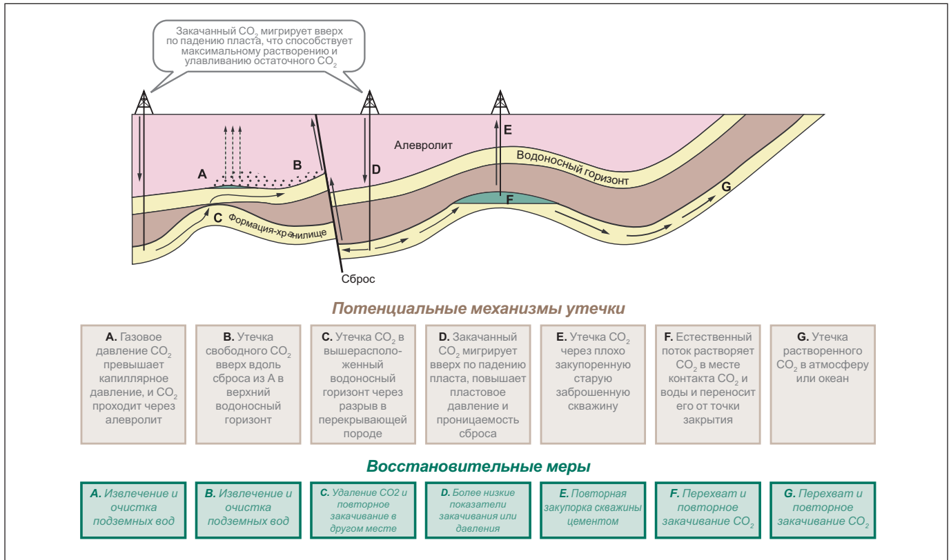
Рисунок ТР.8. Потенциальные маршруты утечки и восстановительные методы для CO 2 , закачанного в соленосные формации. Восстановительная методика будет зависеть от потенциальных маршрутов утечки, обнаруженных в резервуаре. (С разрешения ОЦИТПГ.)
