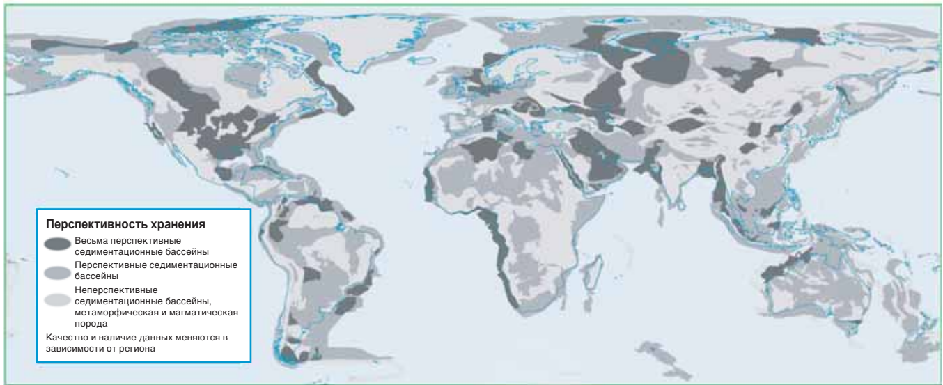
Рисунок TP.2b. Перспективные районы в седиментационных бассейнах, в которых могут быть найдены подходящие соленосные образования, нефтяные или газовые месторождения или угольные пласты. Места для хранения в угольных пластах включены только частично. Перспективность — это качественная оценка вероятности наличия подходящего для хранения места в данном районе на основе имеющейся информации. Этот рисунок следует рассматривать лишь в качестве руководства, поскольку он основан на частичных данных, качество которых может меняться в зависимости от региона и которые могут меняться со временем и с получением новой информации. (С разрешения «Геосайенс Остралия».)
