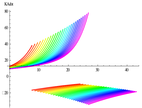
Figure 3.1.A \dot{K}_A : Emax=125-375
