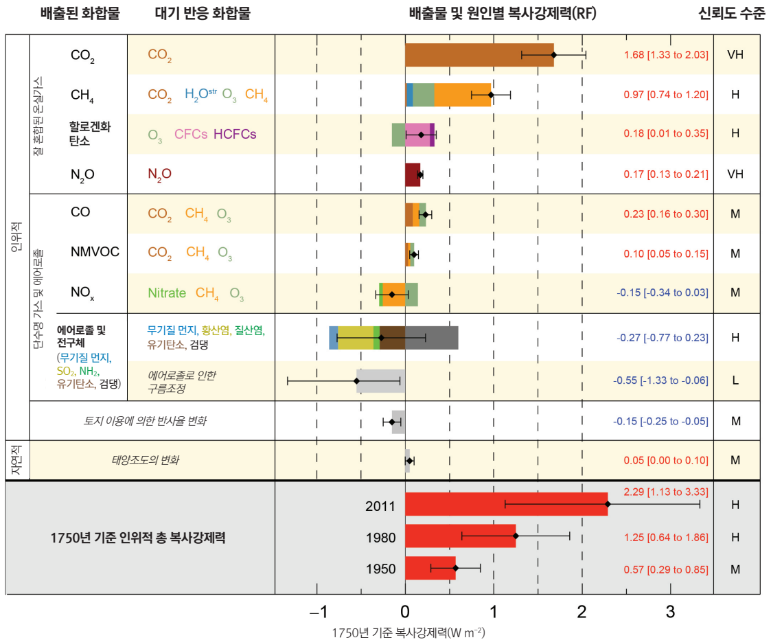
그림 SPM.5: 1750년 대비 2011년의 기후변화의 주요 원인별 복사강제력 추정값과 불확실성. 표시된 값들은 다양한 원인들의 조합을 만들어내는 배출된 화합물과 과정에 따라 구분된 전지구 평균 복사강제력(RF 4 )이다. 순 복사강제력의 최저 추정값은 검정 다이아몬드로 표시하고, 상응하는 불확실성 구간을 함께 제시하였으며, 그 값은 그림의 오른쪽에 신뢰도 수준(VH-매우 높음, H-높음, M-중간, L-낮음, VL-매우 낮음)과 함께 표시하였다. 눈과 빙하 위의 검댕으로 인한 알베도 강제력은 검댕 에어로졸 막대에 포함시켰다. 비행운으로 인한 작은 강제력(비행운 때문에 생긴 권운을 포함하여 0.05 W m^{-2} ), HFC, PFC, SF 6 (총 0.03 W m^{-2} )은 제시하지 않았다. 가스에 대한 농도 기반 복사강제력은 할산하여 유사한 색의 막대그래프로 표현하였다. 화산강제력은 사건 단위로 발생해서 다른 강제력과 비교하기 어렵기 때문에 포함시키지 않았다. 인위적 총 복사강제력은 1750년을 기준으로 3개의 다른 연도에 대해서 제공하였다. 각 물질과 과정에 대한 불확실성 범위 등 보다 기술적인 상세 내용은 TS 보충자료를 참조 {8.5; 그림 8.14~8.18; 그림 TS.6, TS.7}
