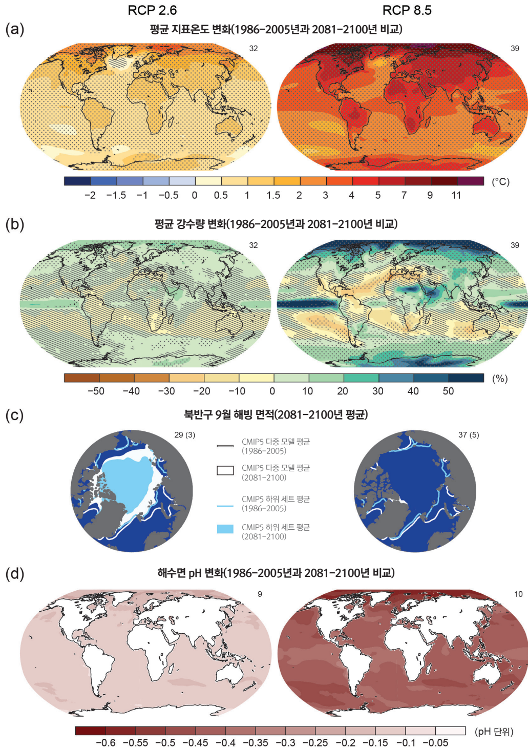
그림 SPM.8: (a) 연평균 지표온도 변화, (b) 연평균 강수량의 평균 변화율, (c) 북반구 9월 해빙면적 (d) 해수면 pH 변화에 대해 CIMP5 다중모델을 이용한 RCP2.6과 RCP8.5 시나리오의 2081~2100년 평균값의 결과를 나타냄. (a), (b)와 (d)의 변화는 1986~2005년 기준기간과 비교하여 표시하였다. 다중모델 평균을 계산하기 위해 사용한 CIMP5 모델의 수는 각 패널의 우측 상단에 표시하였다. 패널 (a)와 (b)의 경우, 선영(hatching) 부분은 다중모델 평균이 자연적 내부변동성(20년 평균에서 자연적 내부변동성의 1 표준편차보다 작은 경우)보다 작은 지역을 표시한다. 점모(stippling) 부분은 다중모델 평균이 자연적 내부변동성(20년 평균에서 자연적 내부변동성의 2 표준편차보다 크다)보다 큰 지역을 표시하고, 모델의 90%가 변화의 경향이 일치하는 경우를 표시한다(박스 12.1). 패널 (c)의 선은 1986~2005년에 대해 모의된 평균이다. 채워진 부분은 금세기 말에 대한 것이다. CIMP5 다중모델 평균은 흰색으로 표시하였고, 기후적 평균상태를 가장 가깝게 재현하는 모델의 서브셋이 예측한 평균 해빙면적(괄호 안에 제시된 모델의 수)과 북극 해빙면적의 1979~2012년 변화경향은 밝은 파란색으로 표시하였다. 보다 상세한 방법론은 TS 보충자료를 참조 (그림 6.28, 12.11, 12.22, 12.29; 그림 TS.15, TS.16, TS.17, TS.20)
